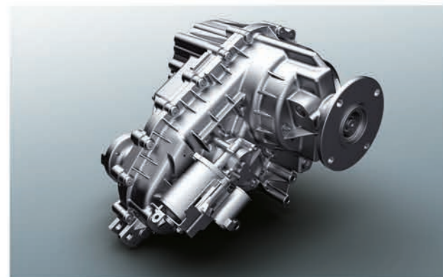
Раздаточная коробка BorgWarner TOD
